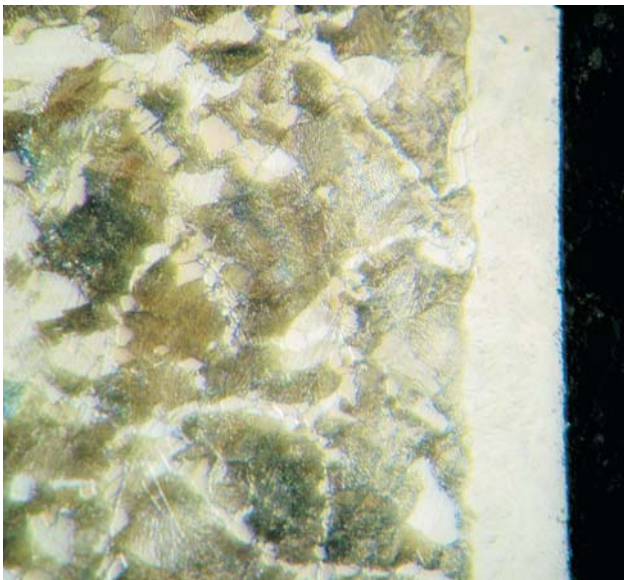
Verbindungsschicht auf einem schmiedeperlitischen Stahl
